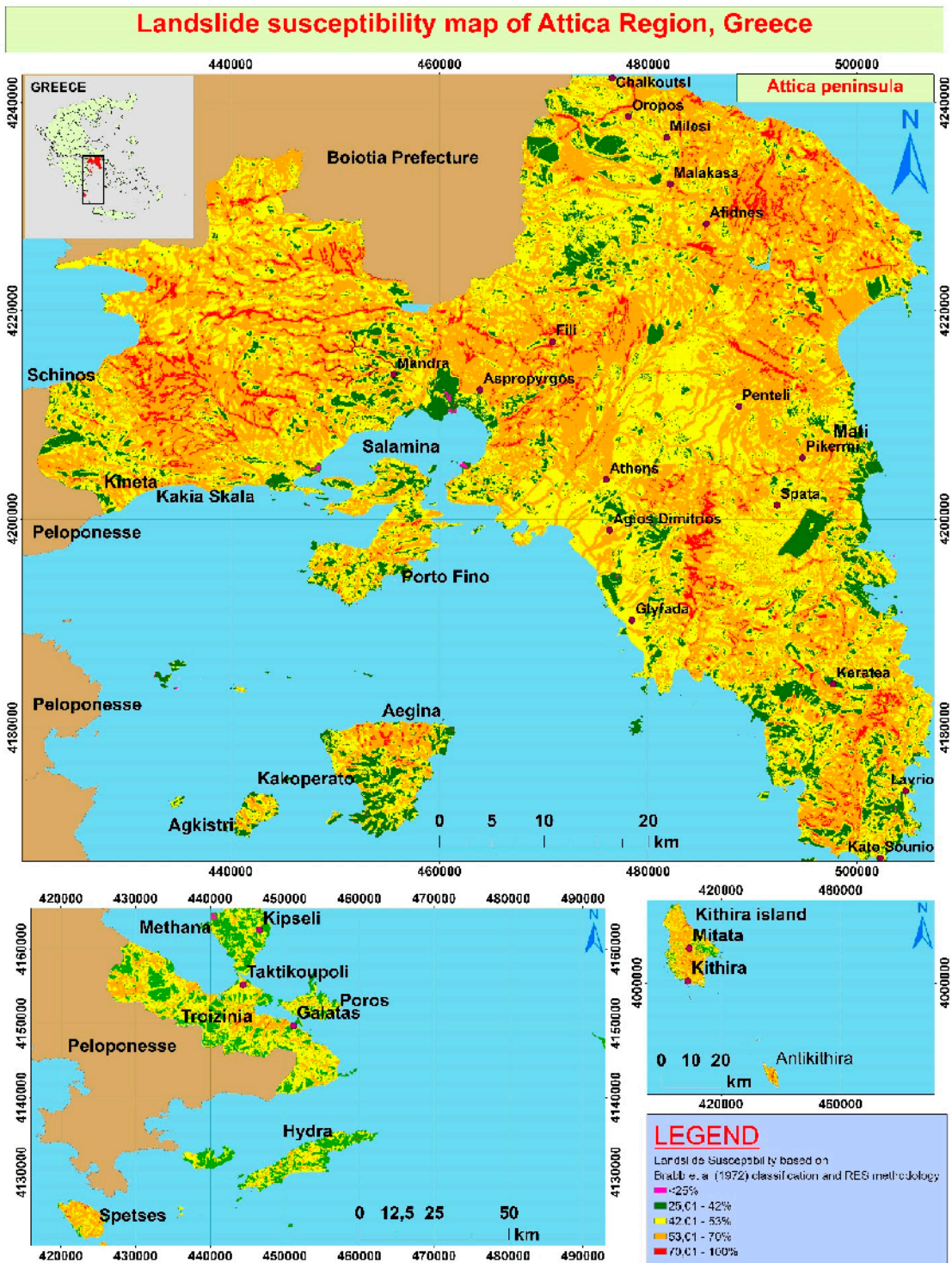
Figura 6.10: Applicazione dell'approccio Rock Engineering System per la mappatura della suscettibilità alle frane nella regione dell'Attica, Grecia.
