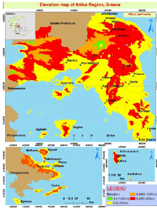
Figure 6.9 Sequenza dei raster tematici
