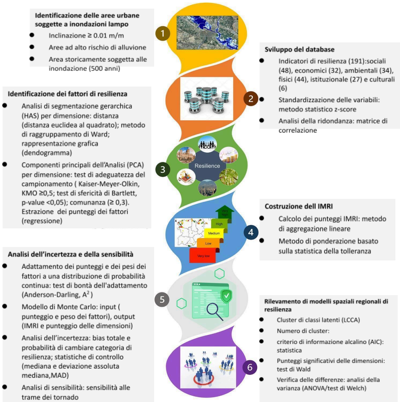
Figura 7.6. Panoramica delle fasi per il calcolo dell'IMRI per quantificare la resilienza alle inondazioni (Aroca-Jiménez et al., 2023).
