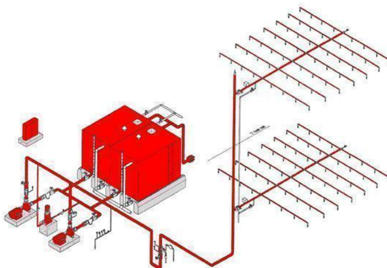
Εικόνα 4.8. Σύστημα ψεκασμού
